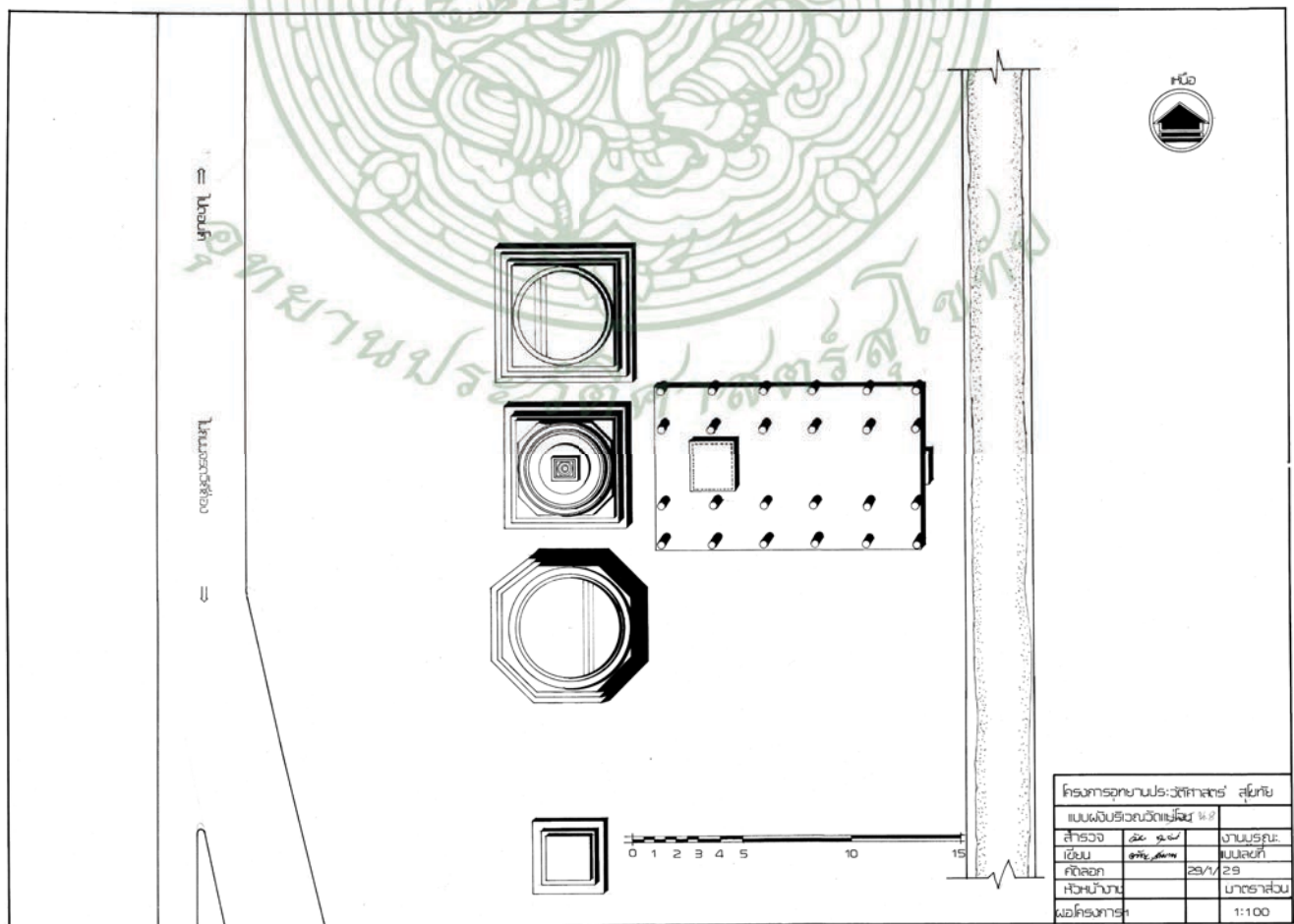
ผังบริเวณโบราณสถานร้าง น.๘
